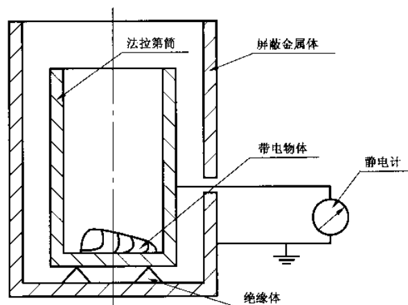
图 A.1 法拉第筒法原理图
